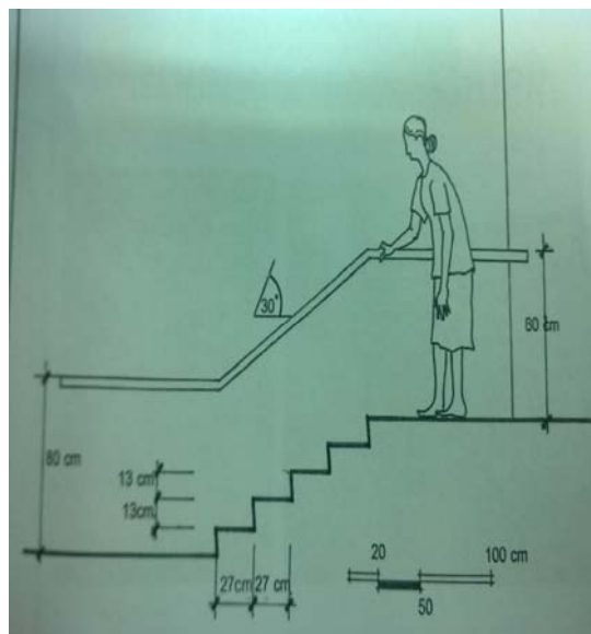
ภาพที่ 2.11 ทางเดินที่มีราวจับ และการปรับปรุงทางเดินให้มีระดับเดียวกัน
