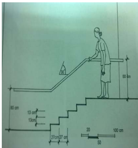
ภาพที่ 3.3 ทางเดินที่มีราวจับ และการปรับปรุงทางเดินให้มีระดับเดียวกัน
