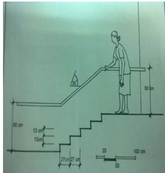
ภาพที่ 11 ทางเดินที่มีราวจับ และการปรับปรุงทางเดินให้มีระดับเดียวกัน
